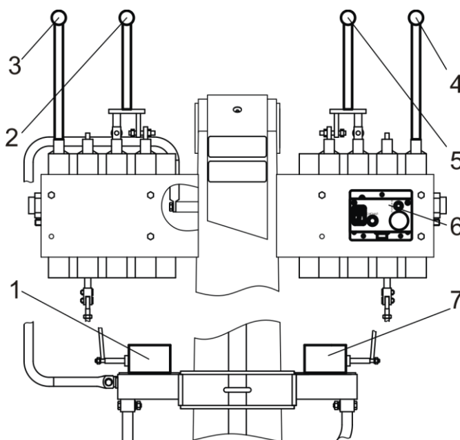
Рисунок 1.2 – Пост управления
